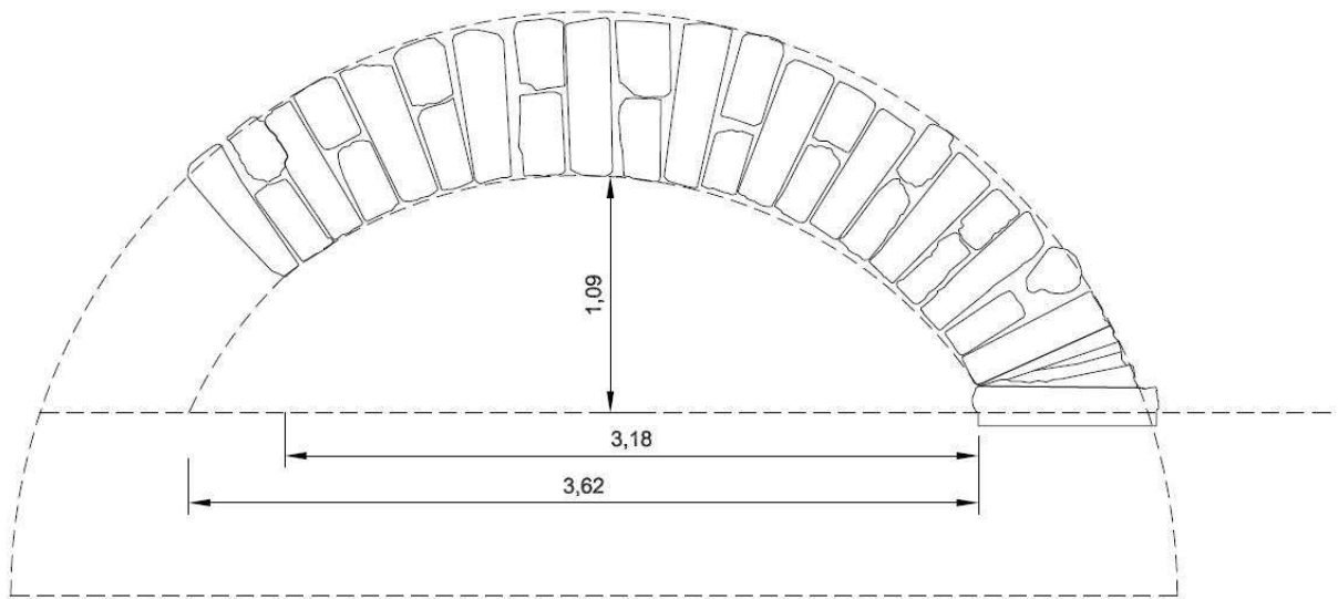
Fig. 152 Dimensiones.
