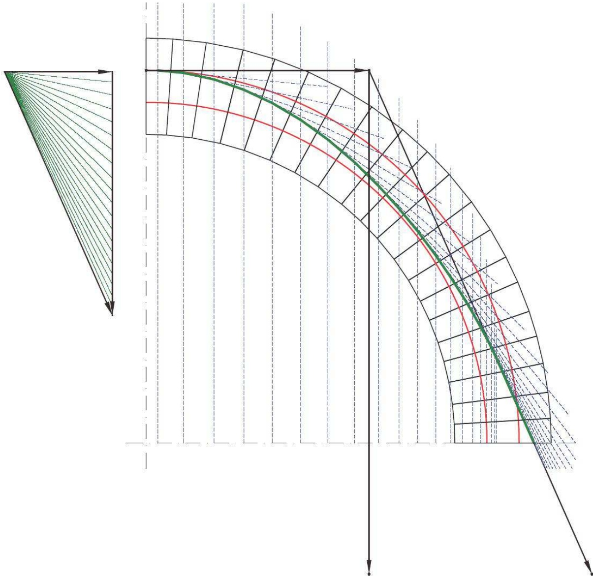
Fig. 156 Análisis gráfico de la estabilidad del arco de medio punto.
