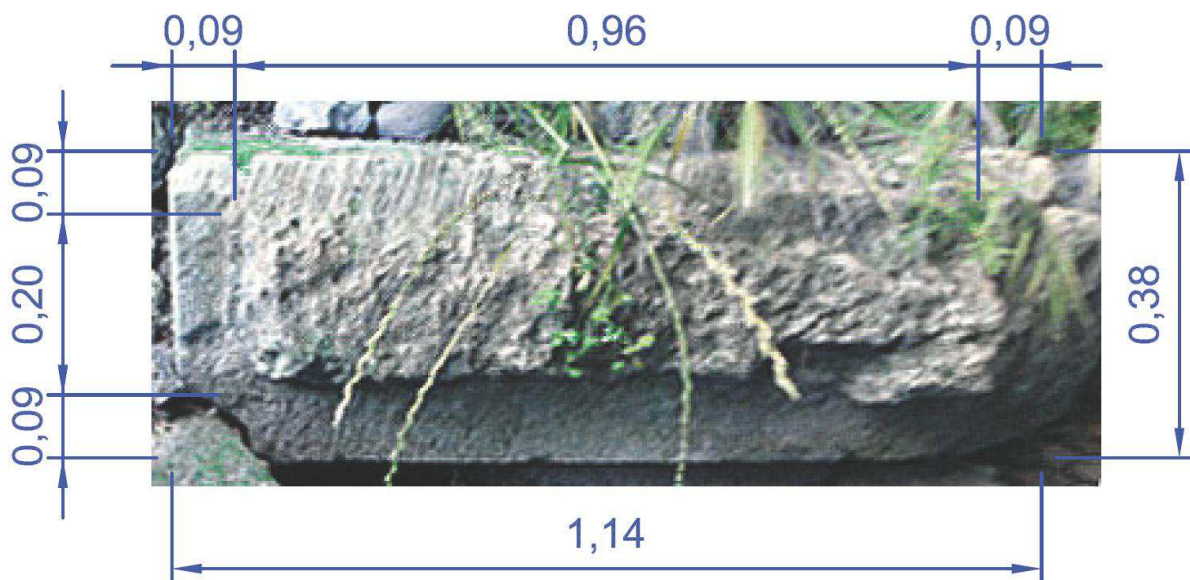
Fig. 66 Dimensiones de un sillar.
